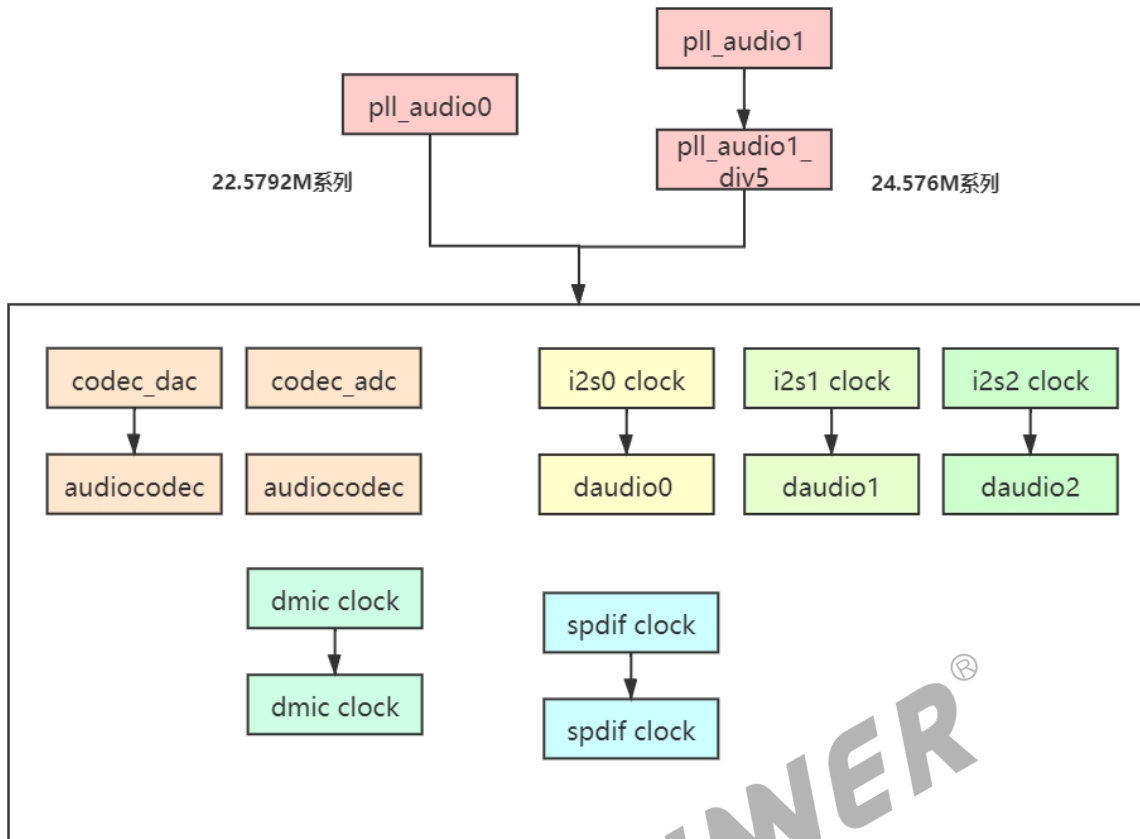
图 2-2: T113s3 时钟源
