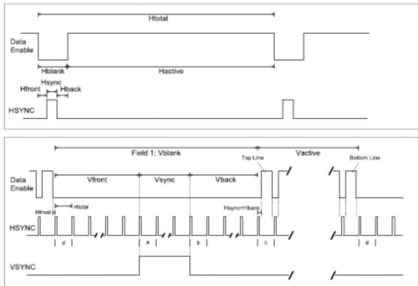
图 6-6: detail timing
